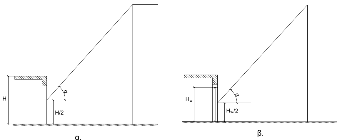
Σχήμα 3.6. Γραφική απεικόνιση της γωνίας θέασης \alpha που σχηματίζουν τα εμπόδια για τον υπολογισμό της σκίασης που προκαλούν σε ένα κατακόρυφο αδιαφανές δομικό στοιχείο ( \alpha ) και σε ένα διαφανές δομικό στοιχείο ( \beta ).
